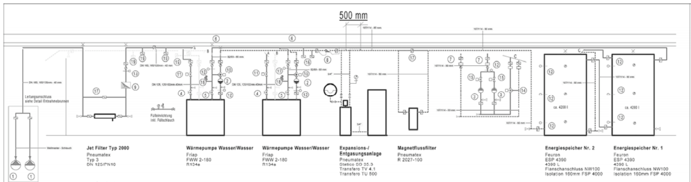
Prinzipschema der FRIAP-Anlage
