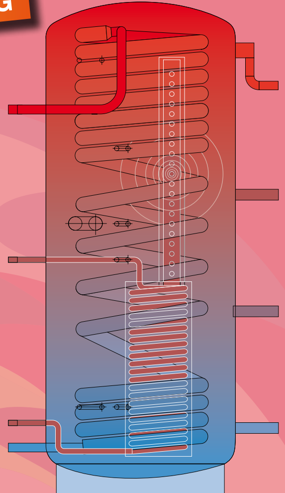
Kombispeicher mit SPIRA Integralboiler Rohmasse: D = 750 mm / H = 1960 mm
