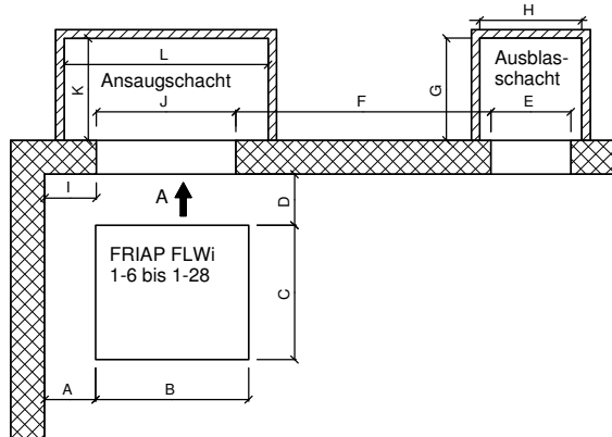
Aussparungsplan Ausblas Rechts
