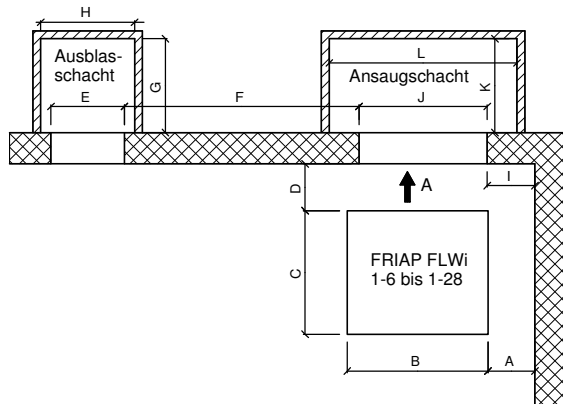
Aussparungsplan Ausblas Links
