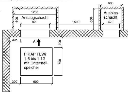
Aussparungsplan Ausblas Rechts
