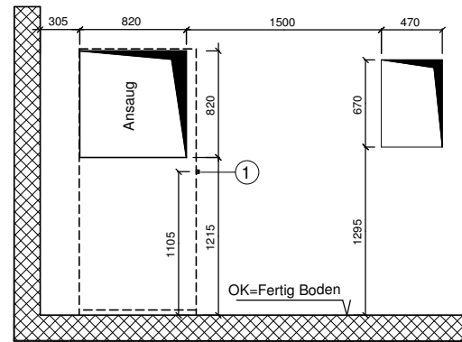
Ansicht A
