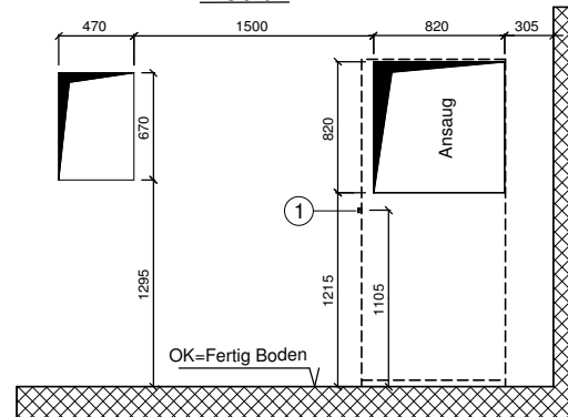
Ansicht A
