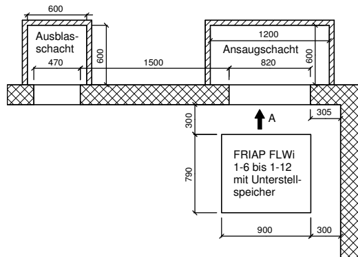
Aussparungsplan Ausblas Links
