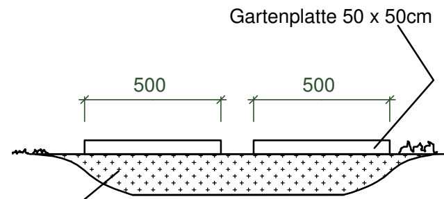
Schnitt
