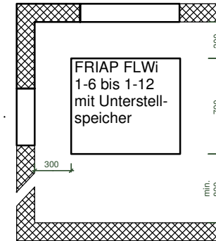
Service-Abstände
