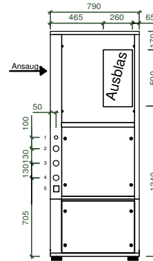
Seitenansicht
